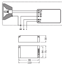
Caractéristiques Osram PTi 1x70/220-240 S
